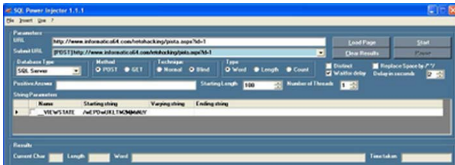
Figura 12. Extracción SQL PowerInjector
