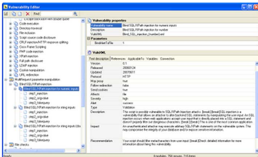
Figura 14: Configuración módulo Blind SQL Injection/Blind XPath Injection para Acunetix Web Vulnerability Scanner4
