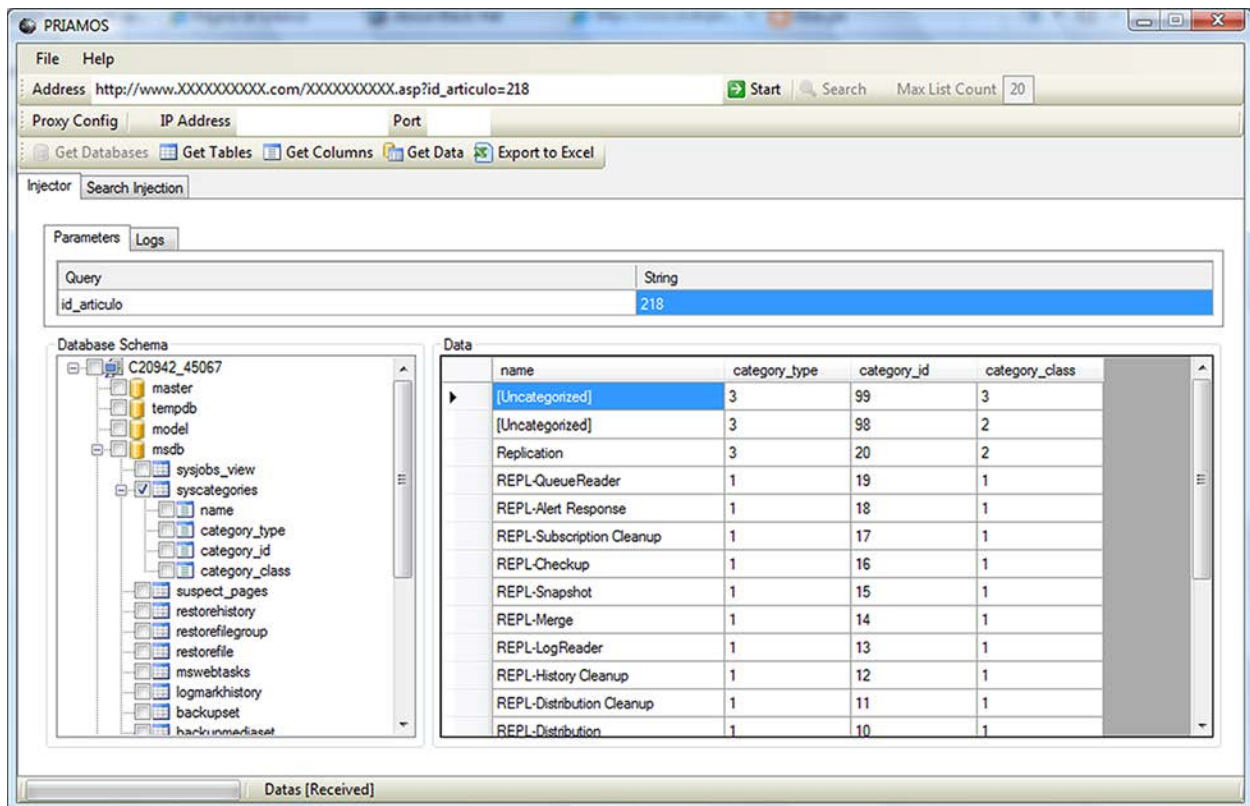
Figura 6. Priamos en funcionamiento
